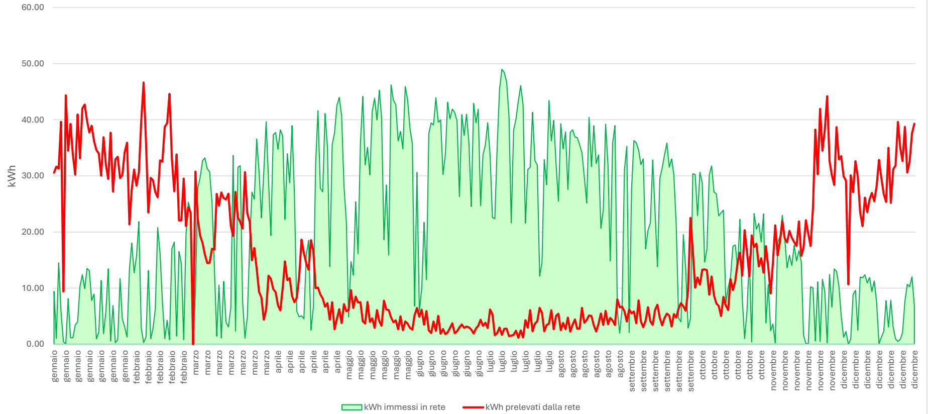
FV Sureggio 2025: energia (kWh) quotidianamente immessa in e prelevata dalla rete (potenza impianto: 9kWp)
