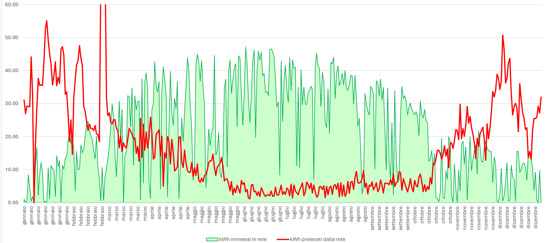
FV Sureggio 2023: energia (kWh) immessa in e prelevata dalla rete (potenza impianto: 9kWp)
